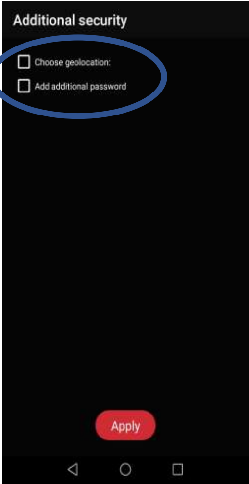
Clon seguro
